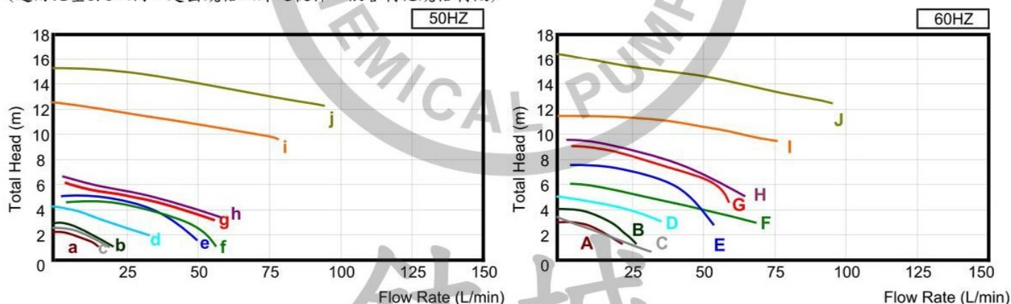
■ 规格表 (0.5HP~10HP×50/60HZ, 清水室温测试)
